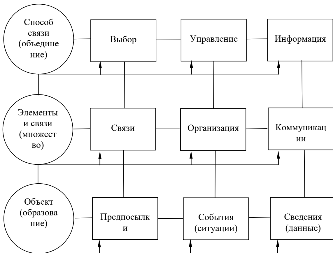
Рис.3.1. Схема взаимосвязи понятий системного исследования
